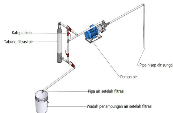
Gambar 1. Desain Geofiltrat Machinery
