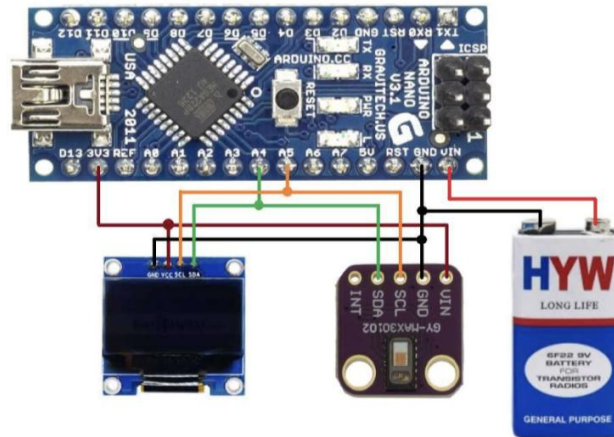
Gambar 1. Diagram pengkabelan alat peraga monitoring kadar oksigen dalam darah.
